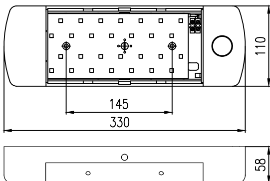
Рисунок - Внешний вид светильника "Омега С*-ДД"
